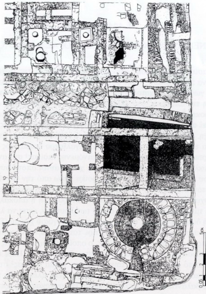
Σχ. 1. Κάτοψη υπάρχουσας κατάστασης νοτιοανατολικής γωνίας του αρχαιολογικού χώρου της (σχέδιο Δ. Καλλιγά, Ζ. Αλ Σααγιάχ).
