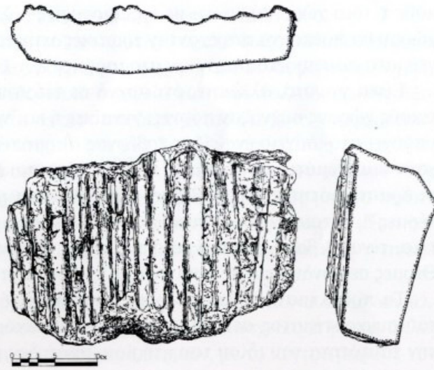
Σχ. 5. Λεπτομέρεια κονιάματος διπλής όψης.
