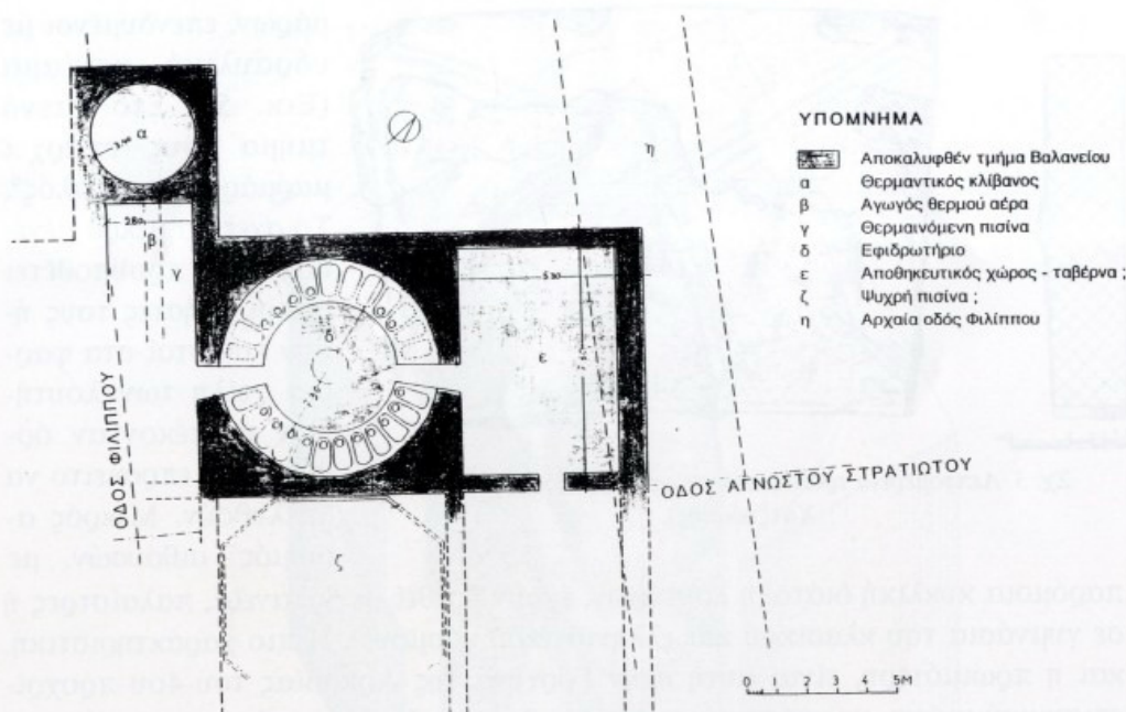
Σχ. 2. Κάτοψη του βαλανείου διακρίνεται η κυκλική, η ορθογώνια αίθουσα, το praefurnium και η ζεστή πισίνα (σχέδιο Δ. Καλλιγά) νότια της κυκλικής αίθουσας και η ψυχρή στα ανατολικά της.
